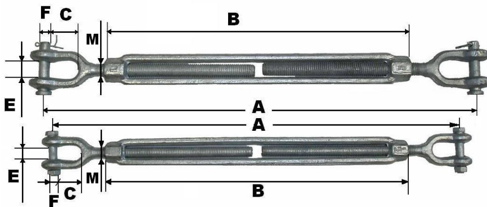
Талрепы вилка-вилка с открытым корпусом
