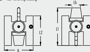
Lasche abgestützt Supported toe
